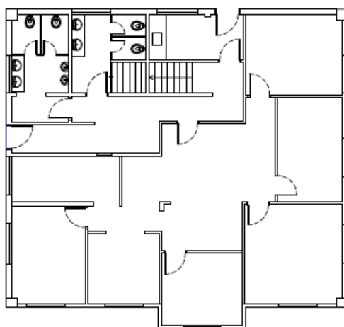
PLANTA TÉRREO
