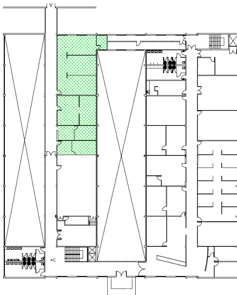
1 PLANTA 1º PAV. ESCALA 1:400
