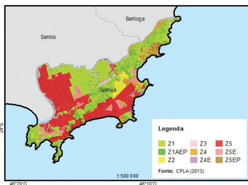
Figura 24 - Mapa do ZEE do Município de Guarujá.
