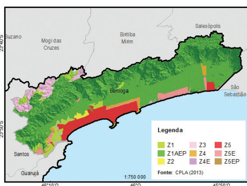
Figura 22 - Mapa do ZEE do Município de Bertioga.
