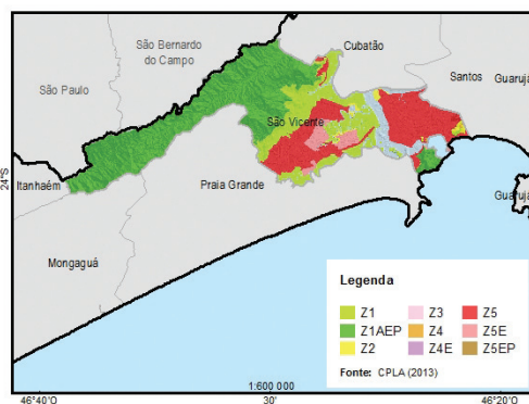
Figura 30 - Mapa do ZEE do Município de São Vicente.
