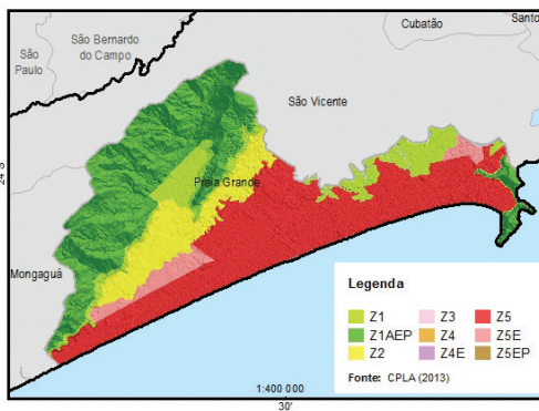
Figura 28 - Mapa do ZEE do Município de Praia Grande.
