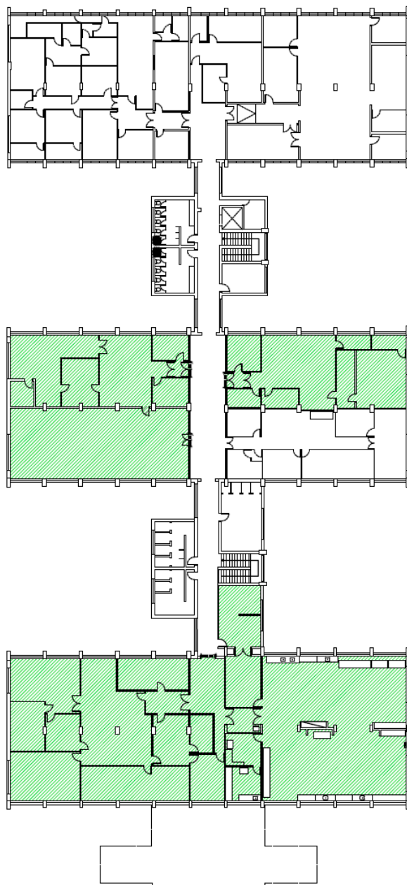
1 PLANTA 2º PAVIMENTO ESCALA 1:850
