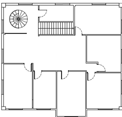
PLANTA 1º PAVIMENTO
