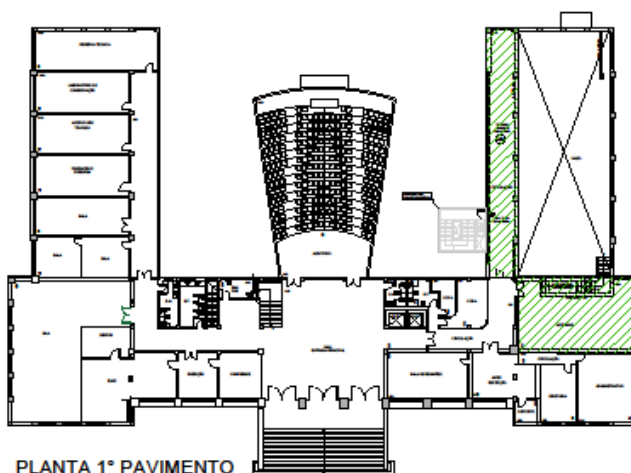
PLANTA 1º PAVIMENTO
